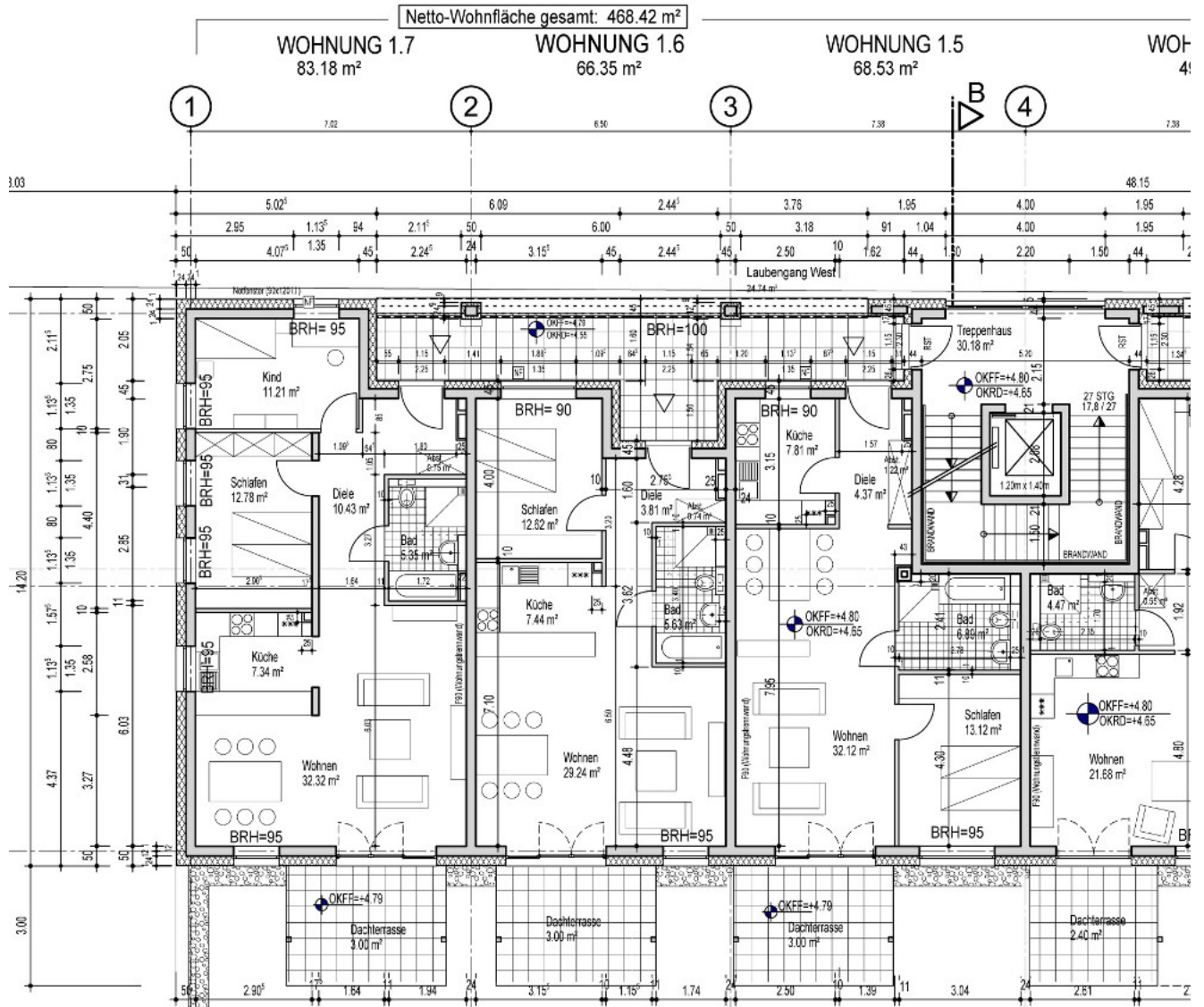
1. OBERGESCHOSS - AUSSCHNITT
